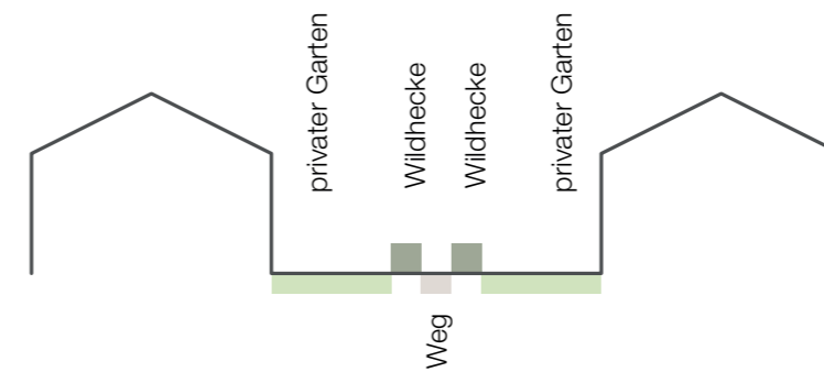
5 Prinzipsschnitt Freihaltebereich
